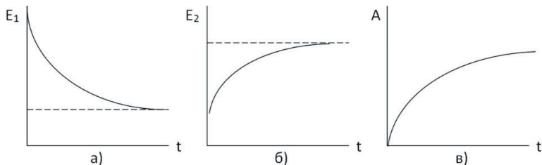
Рисунок 4. Качественный характер динамики показателей E_1 , E_2 , A
