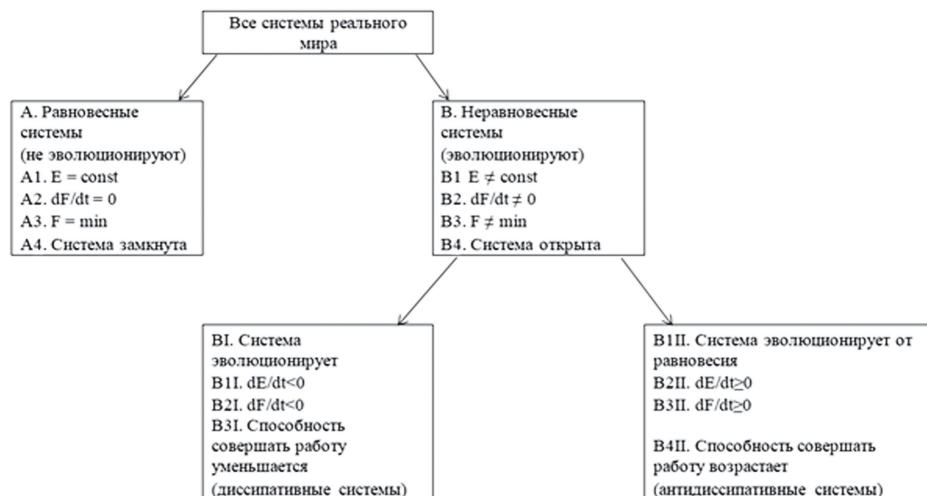
Рисунок 2. Классы неравновесных систем
